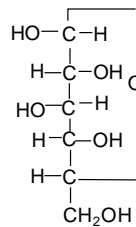
Fig. 4b. \beta -Glucose
