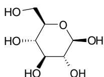
Fig.2a. \beta -D Glucose
