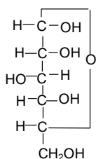
Fig. 4a. \alpha - Glucose
